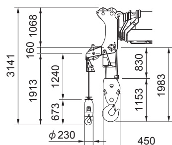
35tonフック
