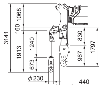
22tonフック
